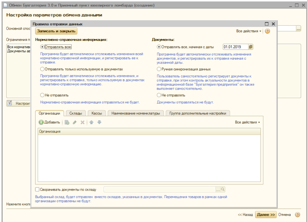
Рис. 19. Правила отправки данных.
