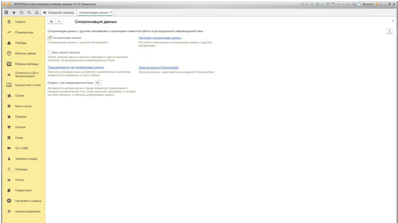
Рис. 2. Синхронизация данных.
