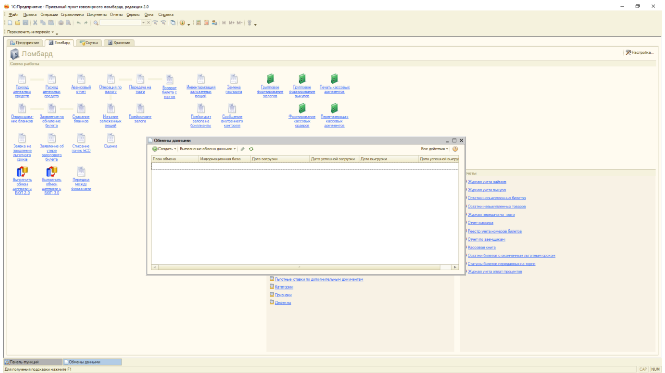
Рис. 14. Обмен данными.
