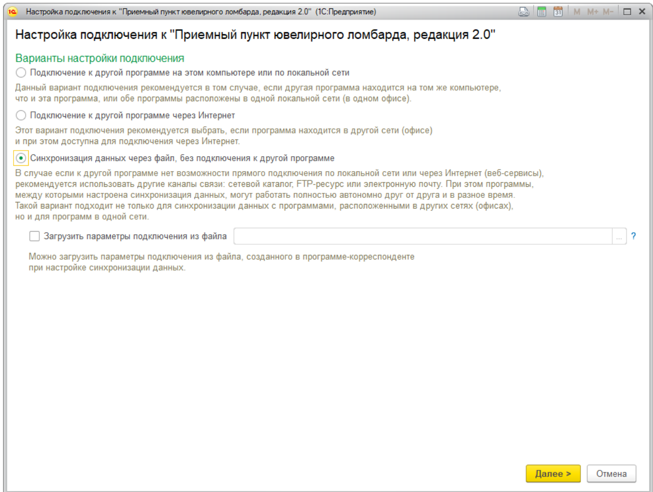
Рис. 5. Настройка подключения.
