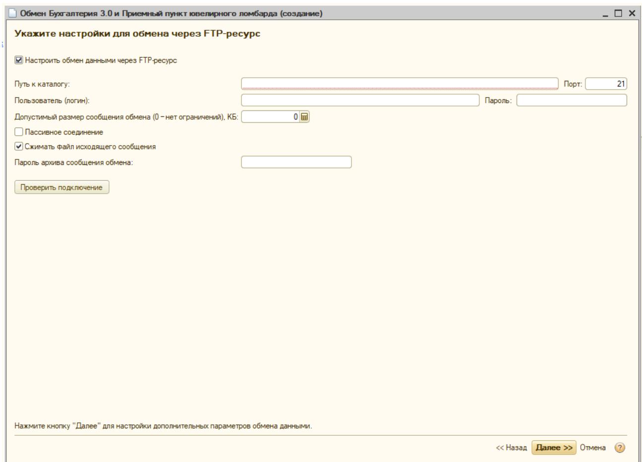
Рис. 17. Настройка обмена через FTP-ресурс.
